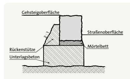
Regelquerschnitt Randeinfassung auf geschalttem Unterlagsbeton
